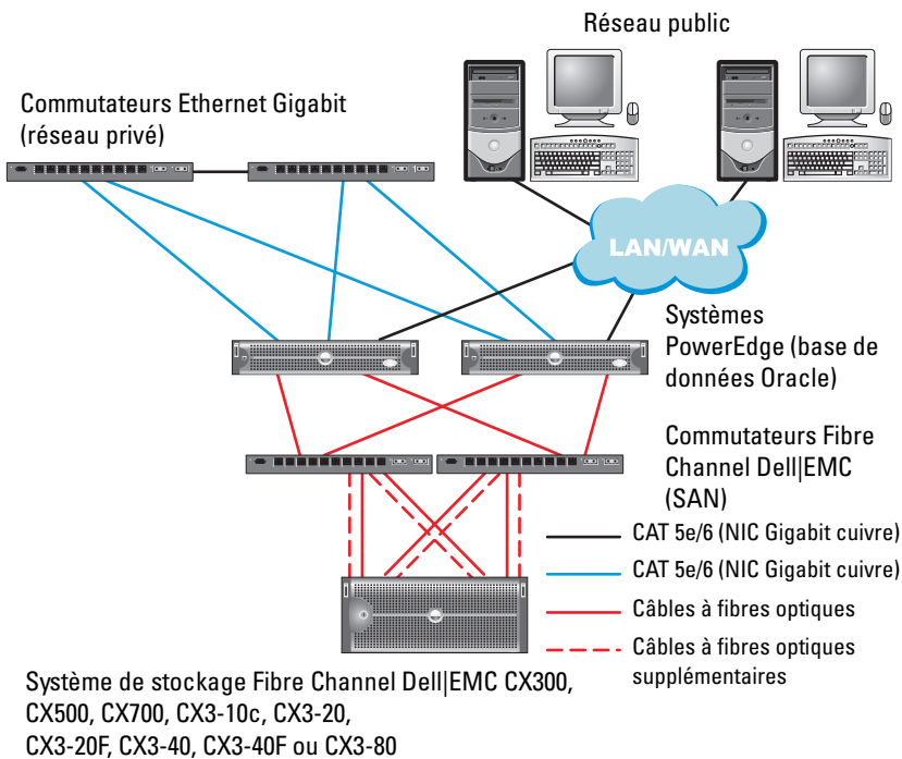
Figure 1-1. Connexions matérielles pour un cluster Fibre Channel relié à un SAN
